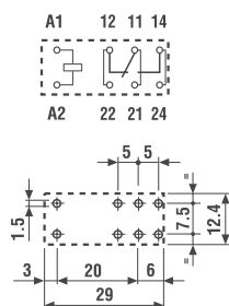
Vista parte inferior Largo de terminal 5.3 mm para CI o zócalos
