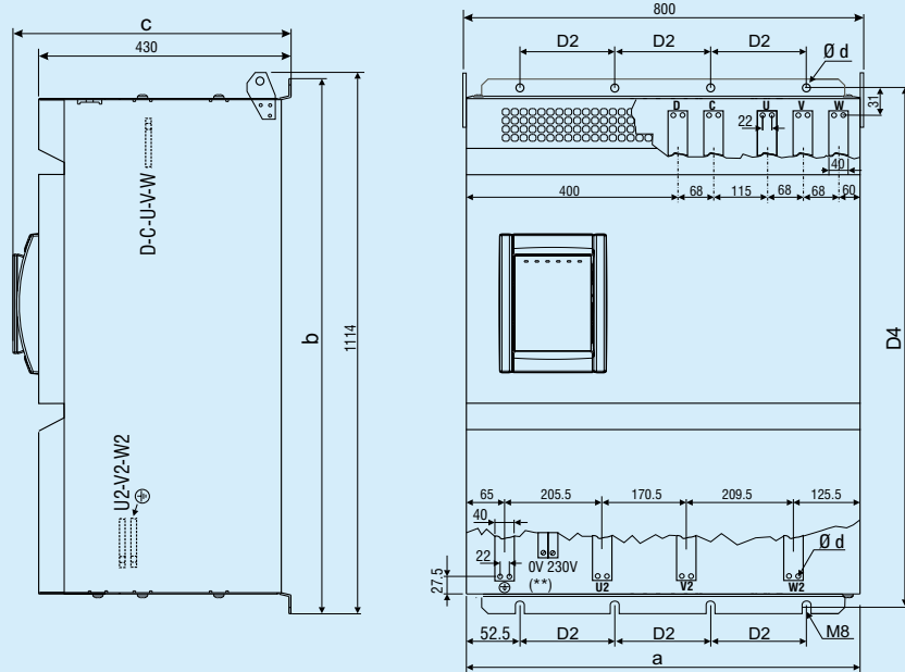
XV y -EV ...-C-IP00 ... XV y -EV ...-CP-IP00
