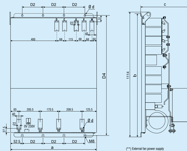
XV y -EV ...-C-IP00 ... XV y -EV ...-CP-IP00
