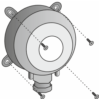
Abb. 2. Montage
